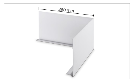
Außenecke: Schlüter®-BARA-FAP/E 90°
