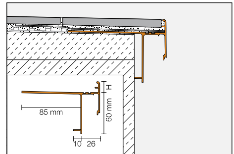
Aufbau mit Schlüter®-DITRA 25 und Schlüter®-BARA-RAKEG
